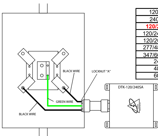
METER SOCKET
